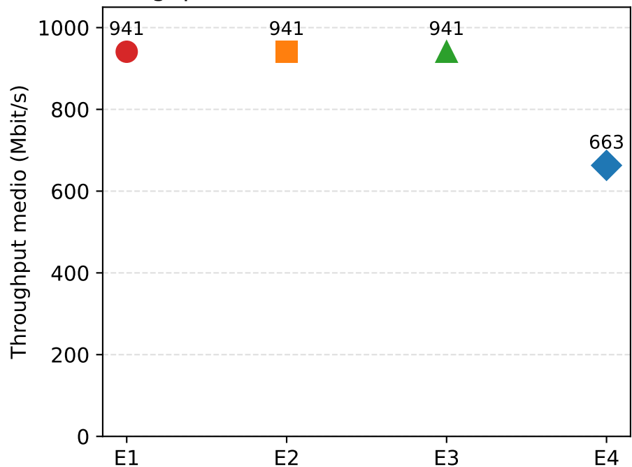
Throughput medio — Baseline (sin límite HTB)
