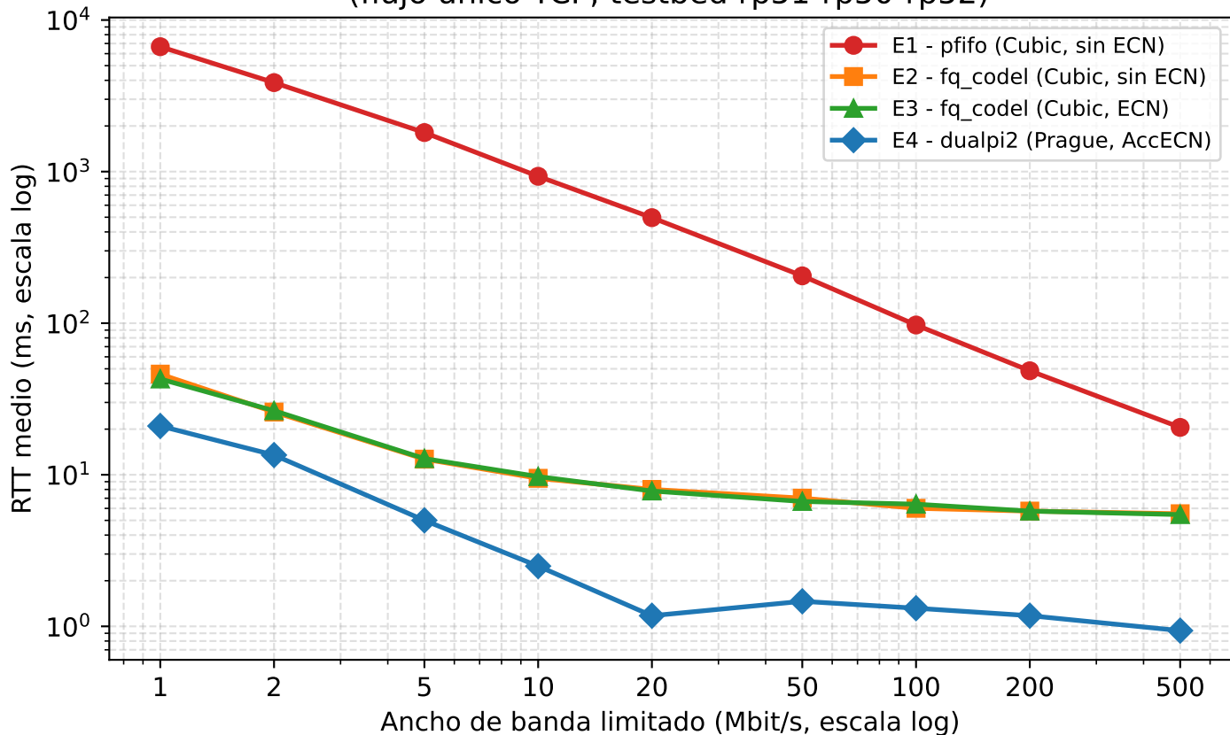
RTT medio por escenario AQM (flujo único TCP, testbed rp51-rp50-rp52)
