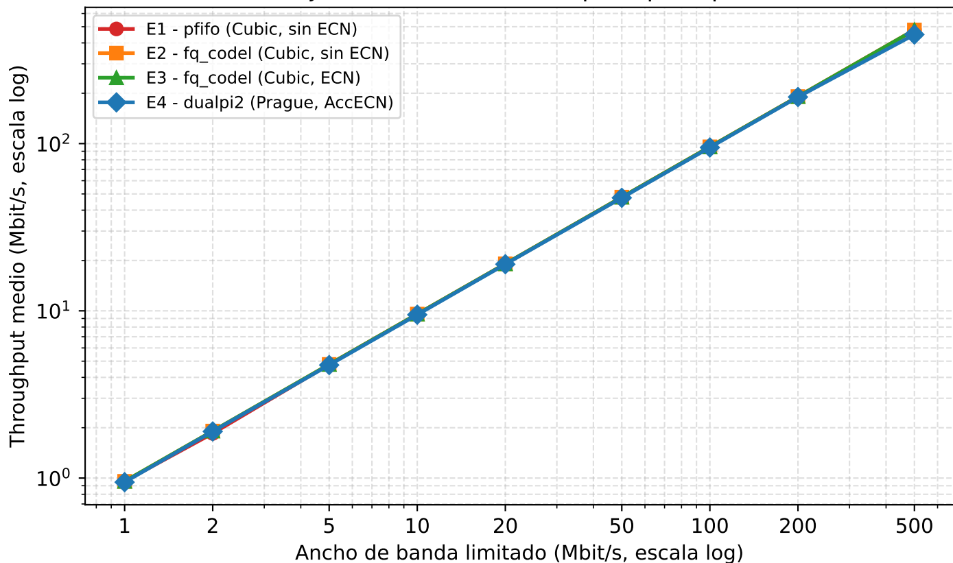
Throughput medio por escenario AQM (flujo único TCP, testbed rp51-rp50-rp52)
