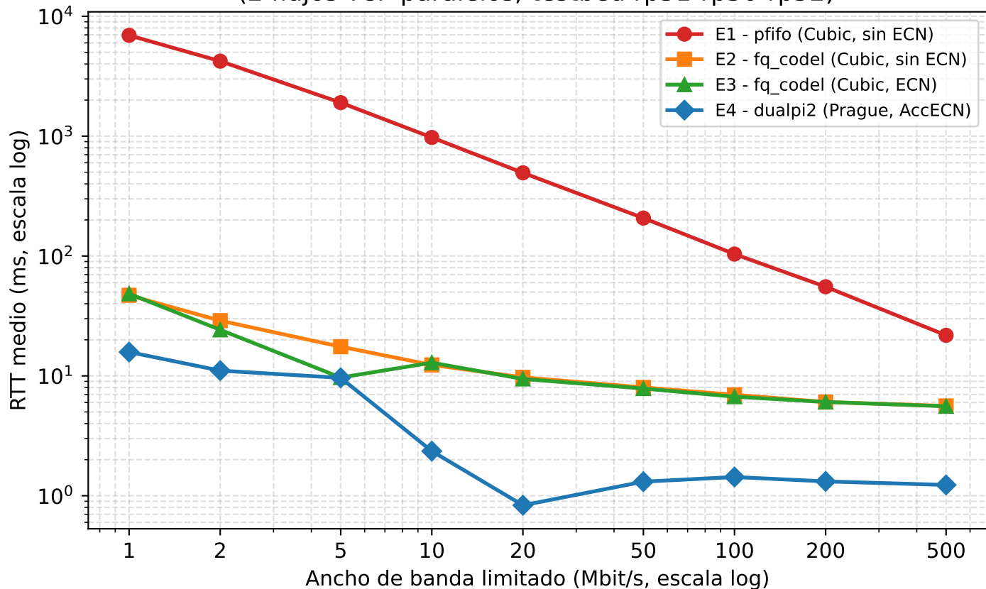
RTT medio por escenario AQM (2 flujos TCP paralelos, testbed rp51-rp50-rp52)
