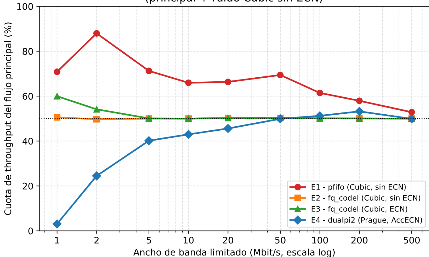
Cuota de throughput del flujo principal sobre el total (principal + ruido Cubic sin ECN)
