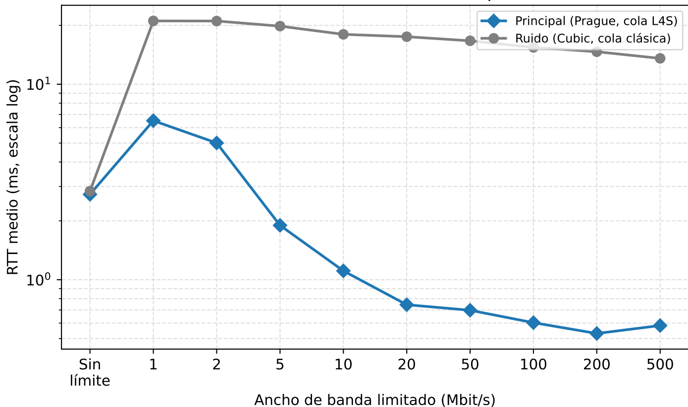
RTT medio por cola en E4 (dualpi2): Prague vs Cubic coexistiendo en la misma disciplina
