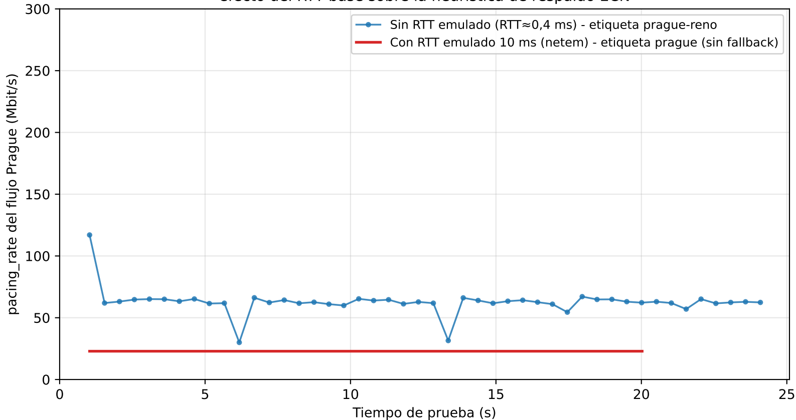
Evolución del pacing_rate de Prague bajo fq_codel (E2, 1xBDP): efecto del RTT base sobre la heurística de respaldo ECN
