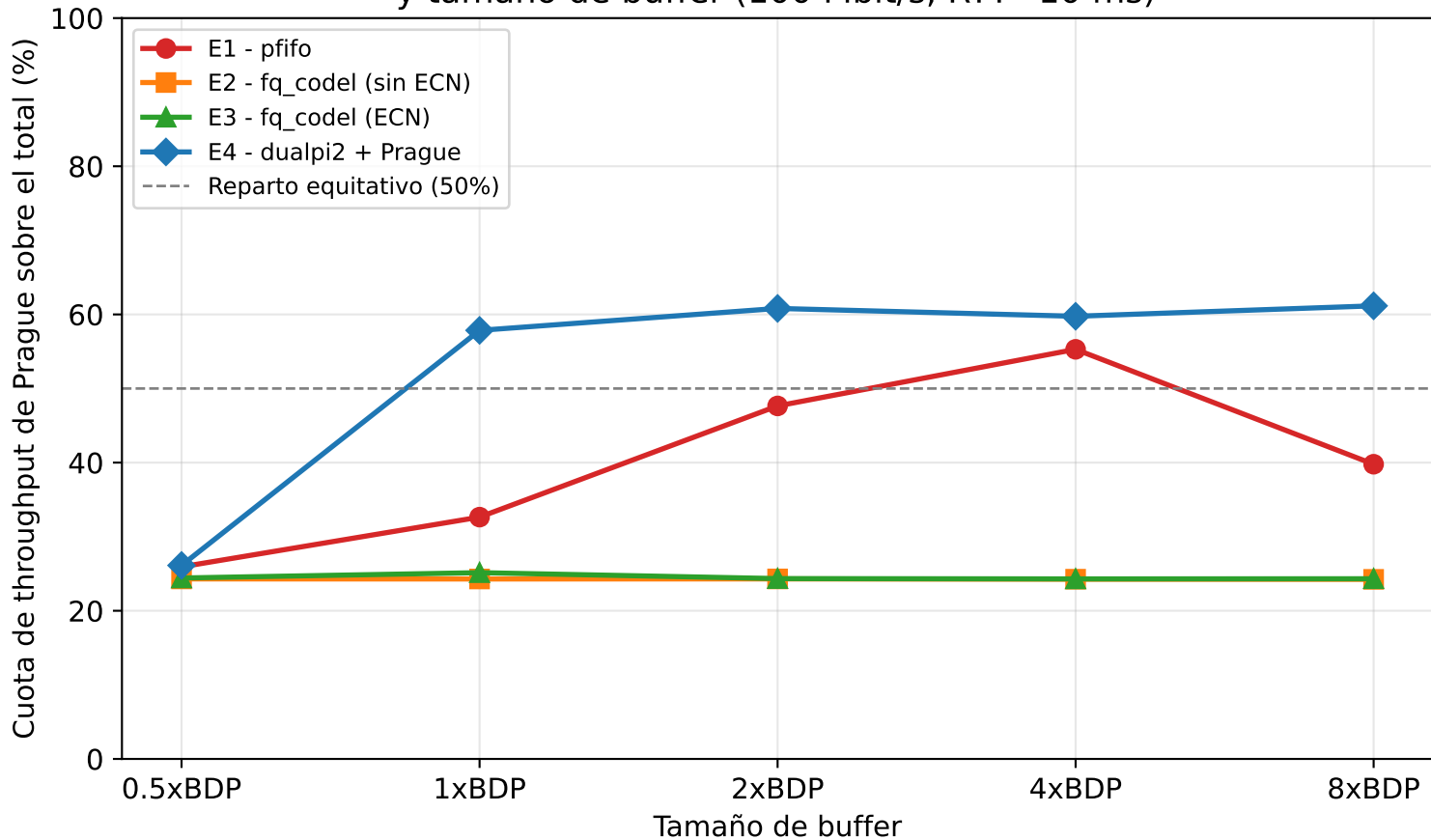
Reparto de throughput Prague/Cubic por escenario AQM y tamaño de buffer (100 Mbit/s, RTT=10 ms)
