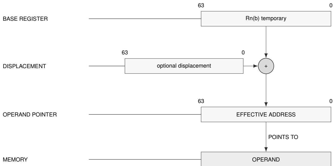
Schema — EXT2 base auto-update
