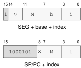
Figure 7-4. EXT2 Descriptor Byte Layouts
