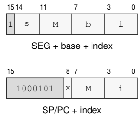
Figure 7-4. EXT2 Descriptor Byte Layouts
