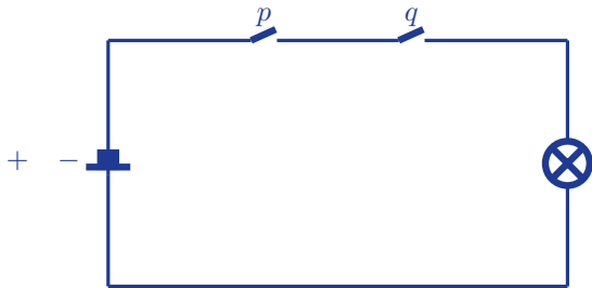
วงจรสวิตช์ไฟฟ้าแบบอนุกรม (AND Operation)
