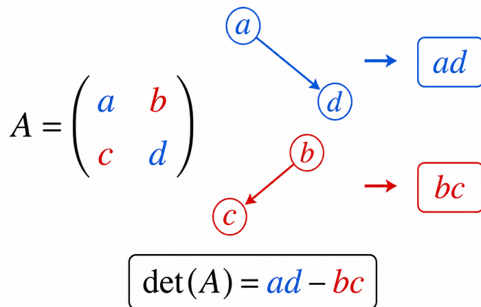
ภาพที่ 20 แผนภาพแสดงดีเทอร์มิแนนต์ของเมทริกซ์ 2 \times 2
