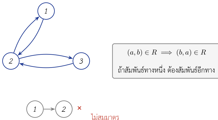
ภาพที่ 15 ความสัมพันธ์สมมาตร (Symmetric Relation) พร้อมลูกศรสองทิศทาง
