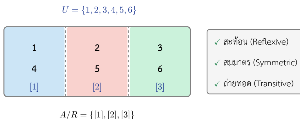
ภาพที่ 18 ความสัมพันธ์สมมูล (Equivalence Relation) แบ่งเซตออกเป็นชั้นสมมูล
