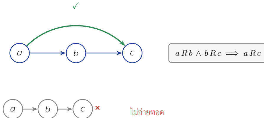
ภาพที่ 17 ความสัมพันธ์ถ่ายทอด (Transitive Relation) แสดงลูกโซ่ a \rightarrow b \rightarrow c
