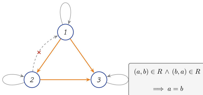
ภาพที่ 16 ความสัมพันธ์ปฏิสมมาตร (Antisymmetric Relation) พร้อมลูกศรทิศทางเดียว
