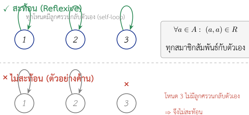
ภาพที่ 14 ความสัมพันธ์สะท้อน (Reflexive Relation) พร้อมลูกศรวน (loops) แสดง (a, a)
