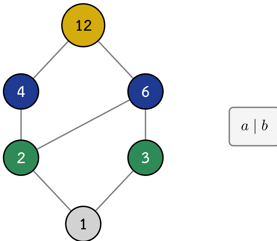
ภาพที่ 19 ไดอะแกรมฮัสเซอ (Hasse Diagram) แสดง Partial Order จากความสัมพันธ์หารลงตัว
