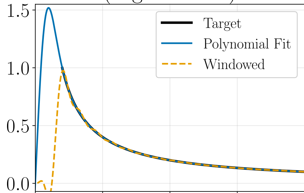
Optimal + Window (deg 101+102)
