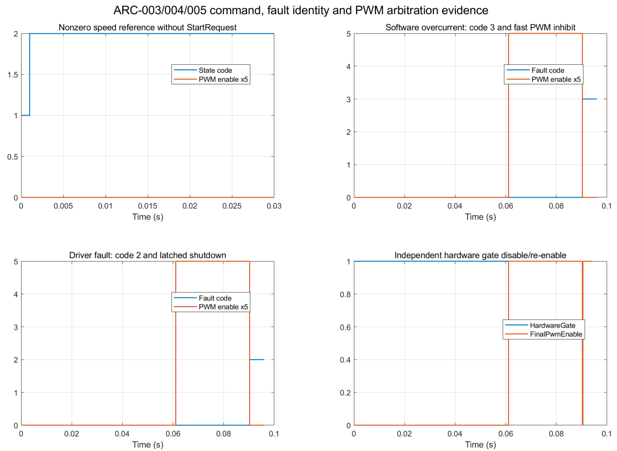
图 6 ARC-003-005 无启动、过流、驱动故障和 HardwareGate 专项证据
