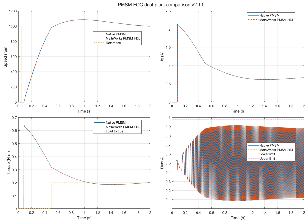
图 7 两个 PMSM 被控对象的速度、 I_q 、转矩和 Duty A 曲线
