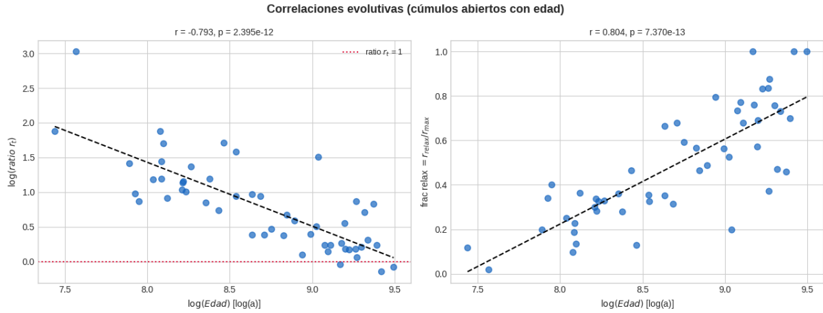
Figura 4.9: Diagramas de dispersión \log(\text{ratio } r_t) vs. \log(\text{años}) (izquierda) y f_{\text{relax}} vs. \log(\text{años}) para la submuestra de 52 cúmulos abiertos con edad disponible, con regresiones lineales. La línea horizontal \text{ratio } r_t = 1 en el panel izquierdo marca el umbral de relajación al radio de marea.
