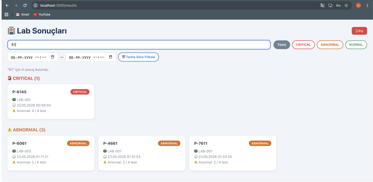
Şekil 5: Kısmi ID ile arama
