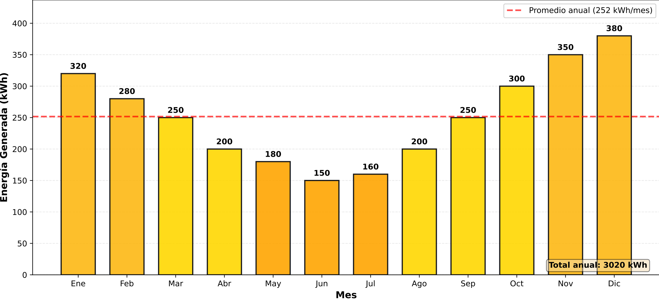
Generación Mensual Estimada - Caso de Prueba (8 paneles, 2.8 kW)
