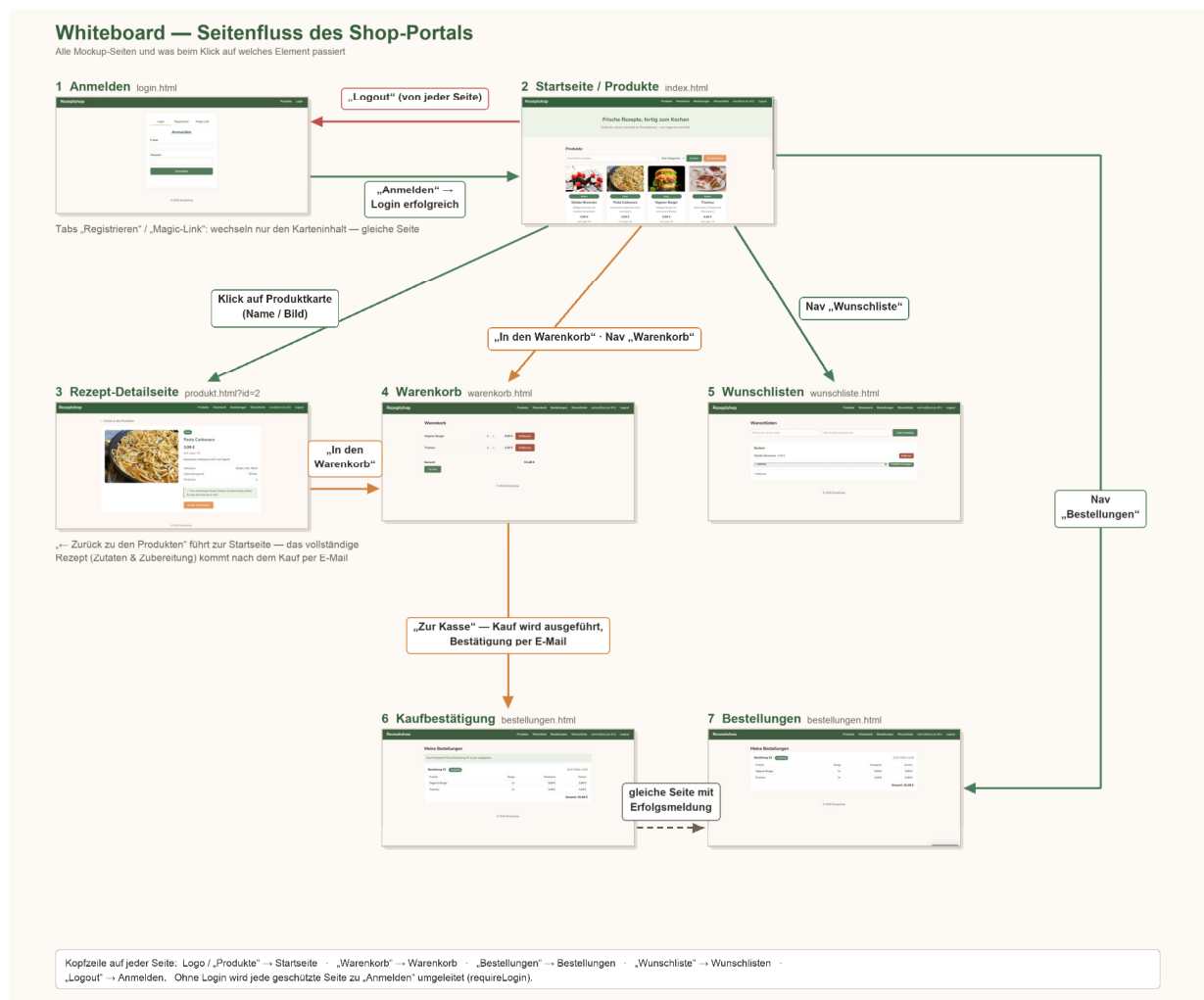
Abbildung 13: Whiteboard Shop-Portal: alle Seiten mit Klick-Zielen und Übergängen
