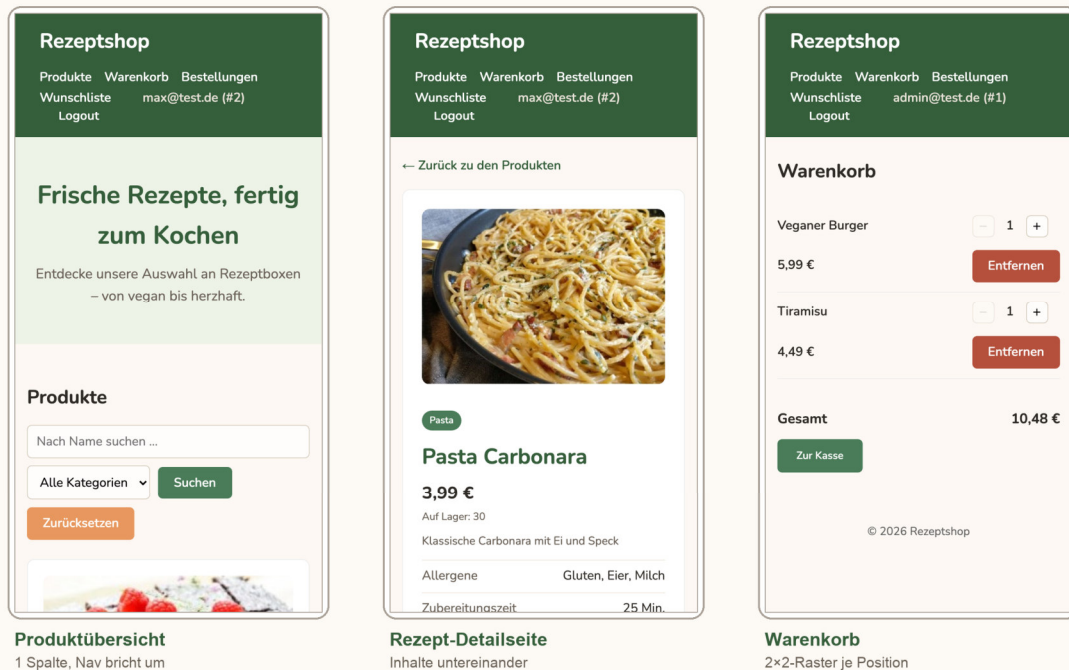
Abbildung 15: Hochformat-Ansichten (390 px): Produktübersicht, Rezept-Detailseite und Warenkorb
