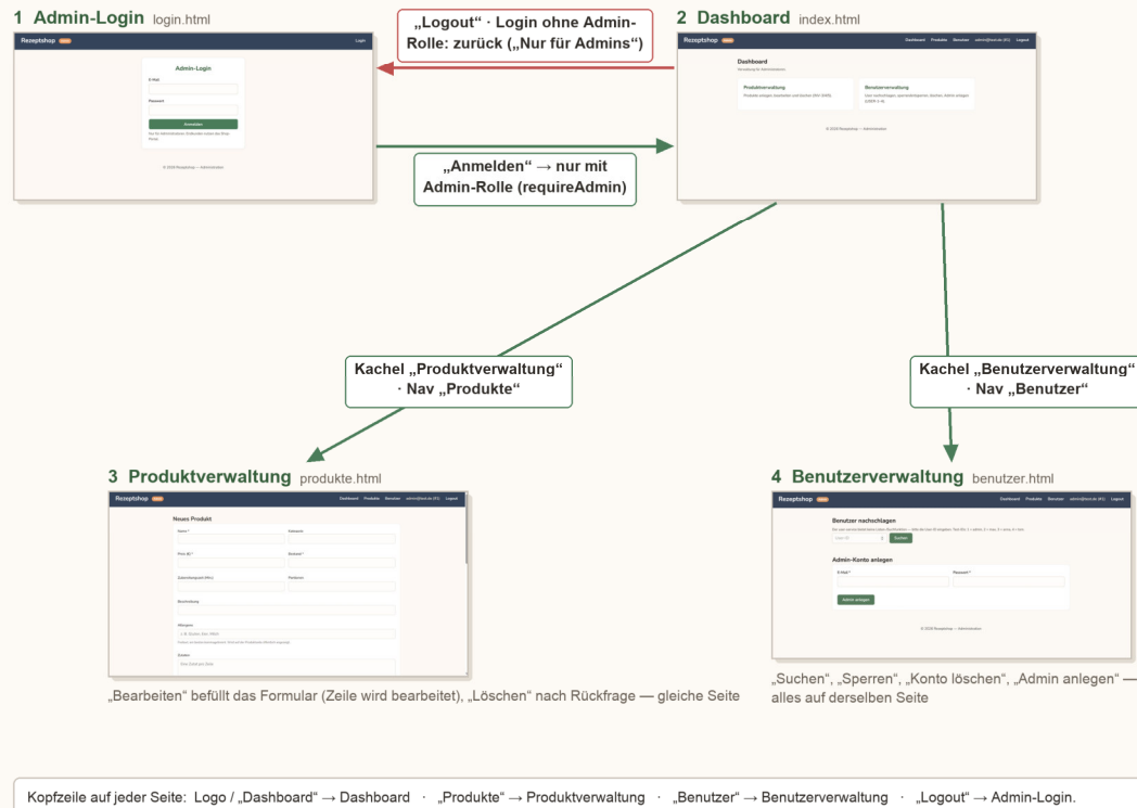
Abbildung 14: Whiteboard Admin-Portal: Login mit Rollenprüfung, Dashboard und Verwaltungsseiten
