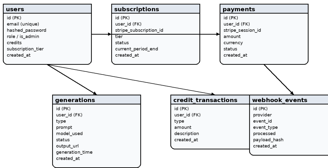
AI Studio Pro - Database ER Diagram
