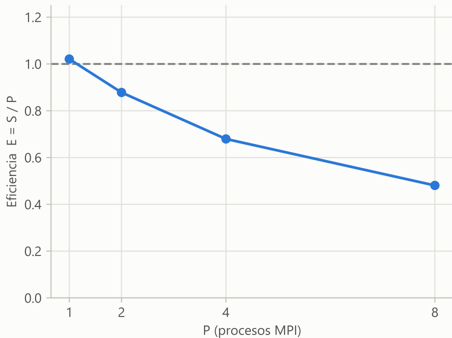
Eficiencia de mpi_v2 — \pi con N = 10^9
