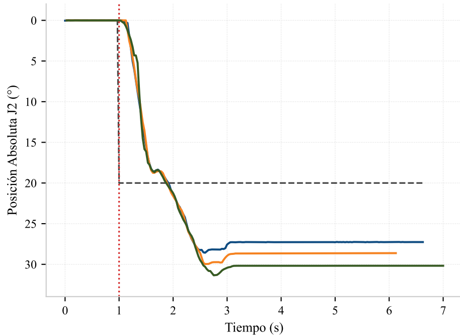
Posición Articulación 2 (Fémur)
