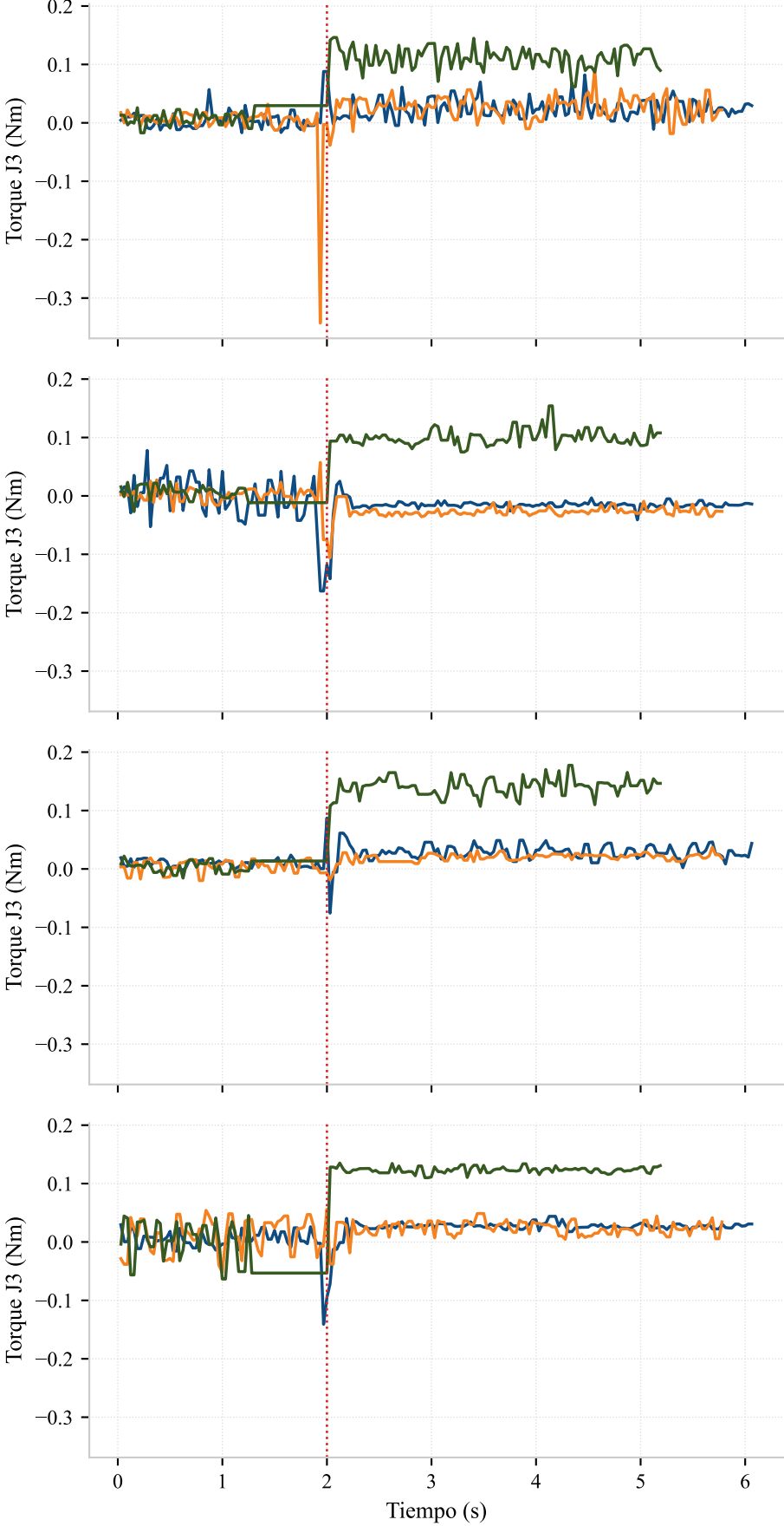
Torque Articulación 3 (Tibia)
