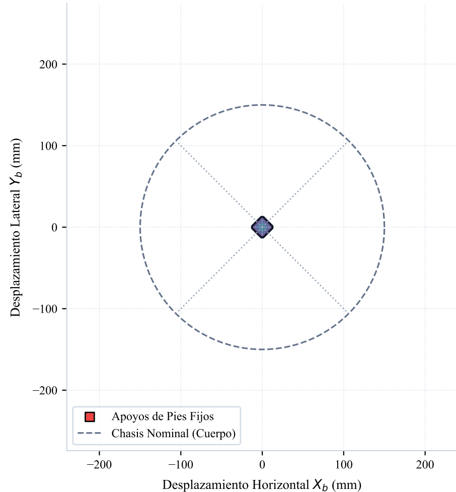
(a) Espacio de Trabajo Horizontal (Plano X_b - Y_b a Z_b = 0 )
