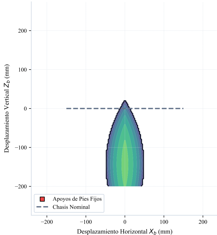
(b) Espacio de Trabajo Sagital (Plano X_b - Z_b a Y_b = 0 )
