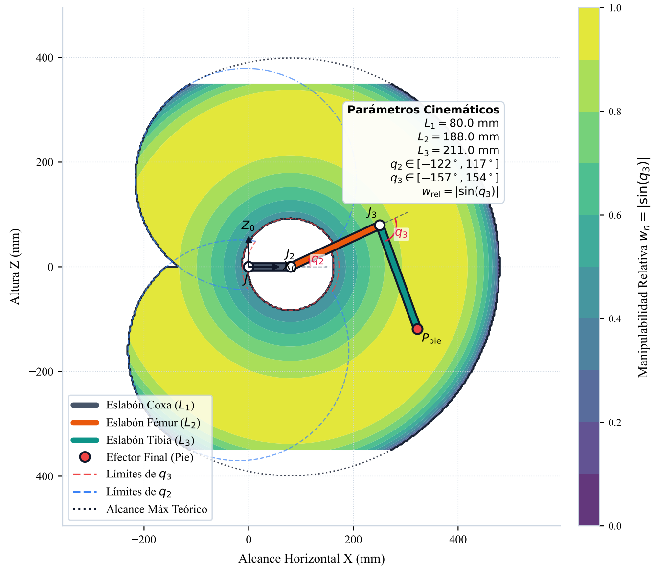
(b) Envoltura de Trabajo Sagital (Plano X-Z)
