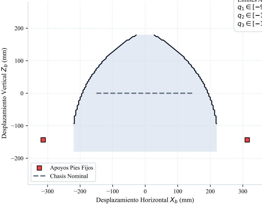
(c) Proyección en el Plano Sagital X_b - Z_b
