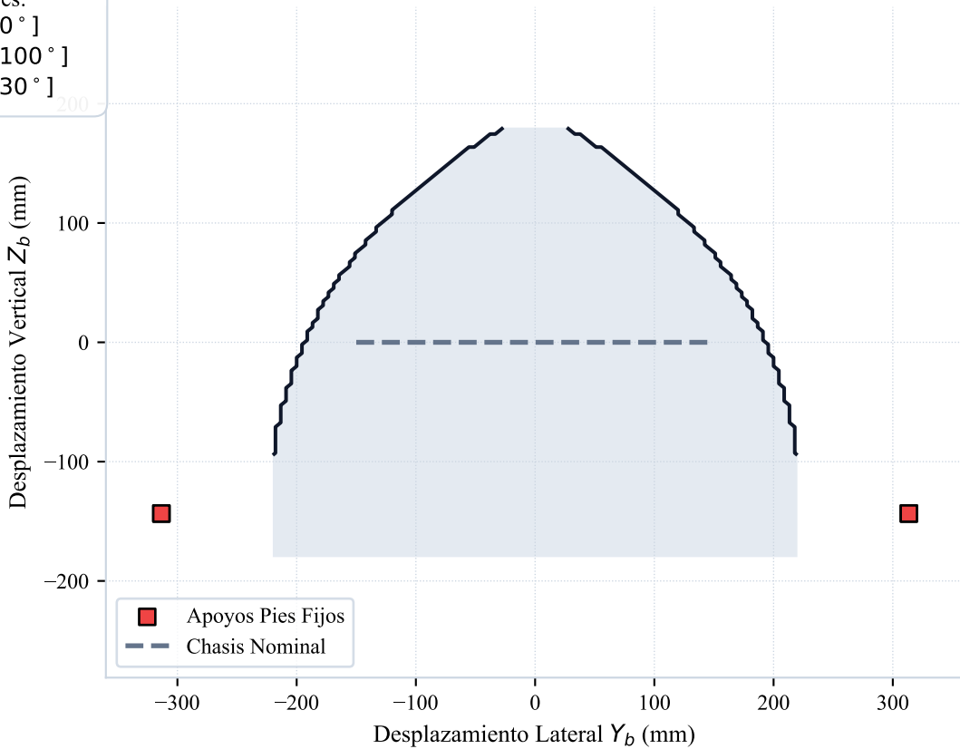
(d) Proyección en el Plano Frontal Y_b - Z_b
