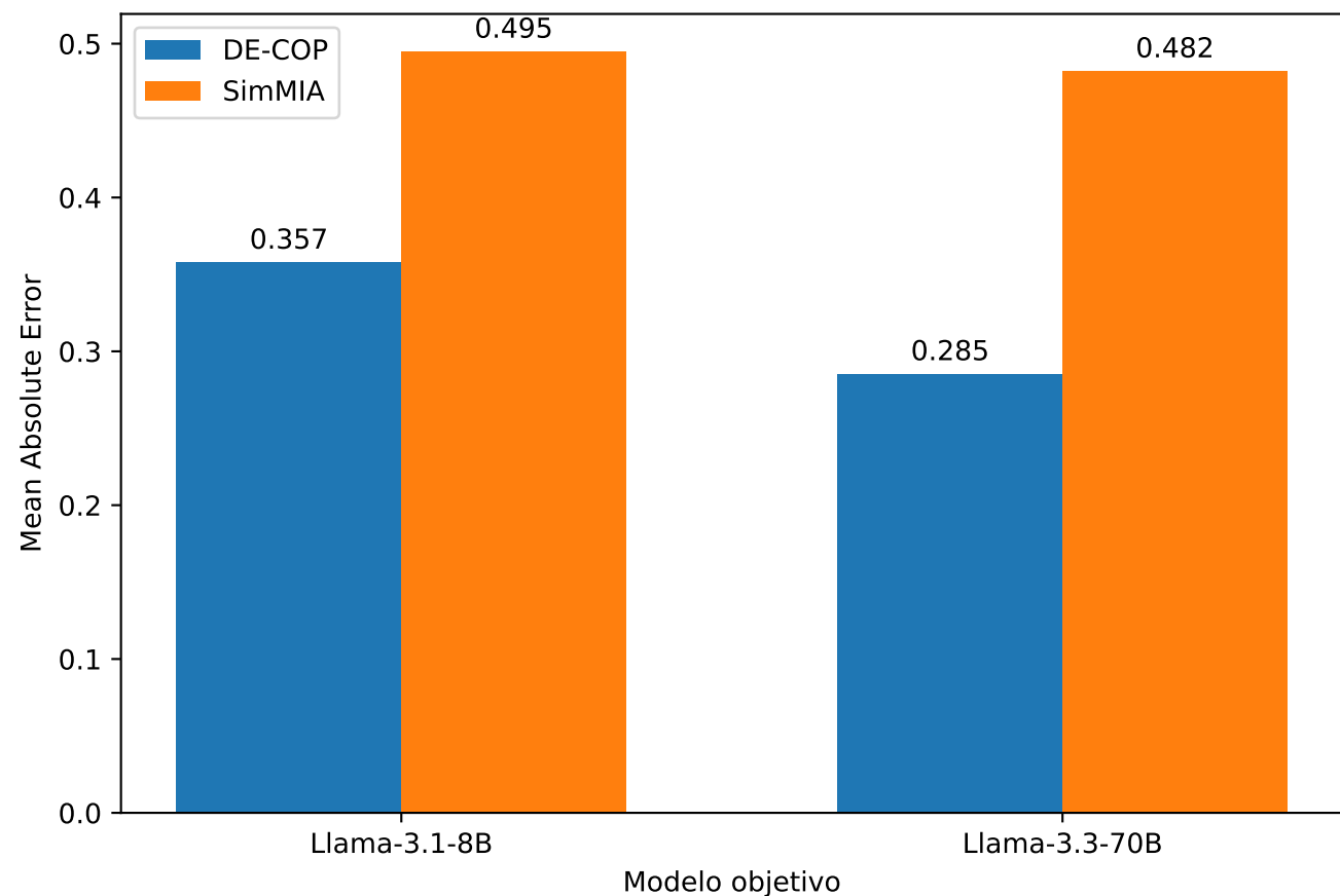
Error absoluto medio sobre BookTecton
