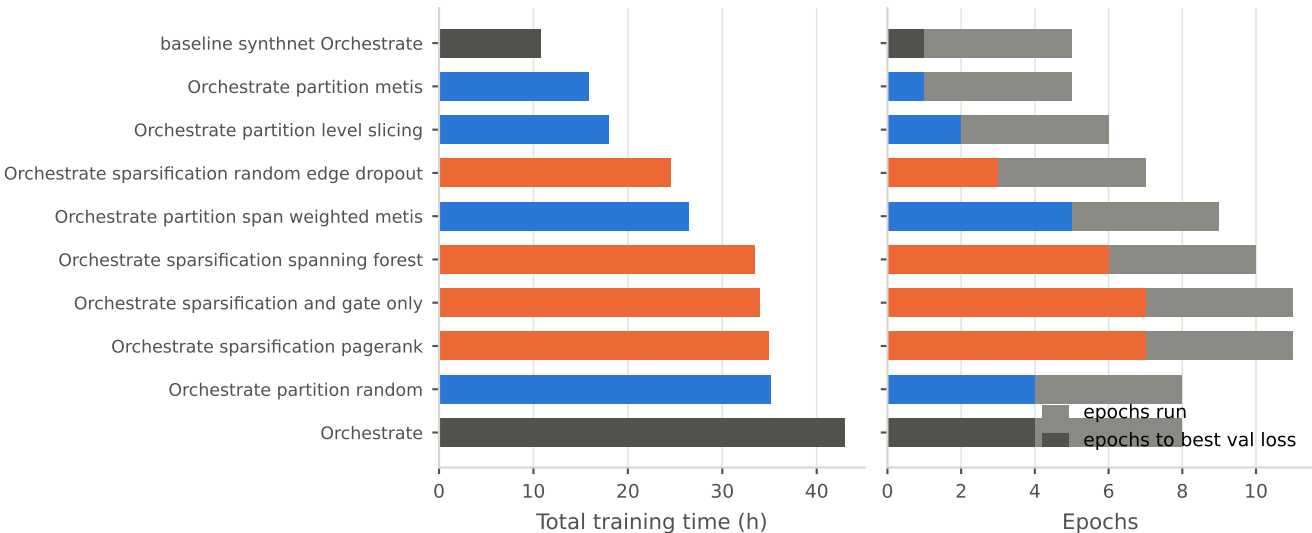
Wall-clock per run
