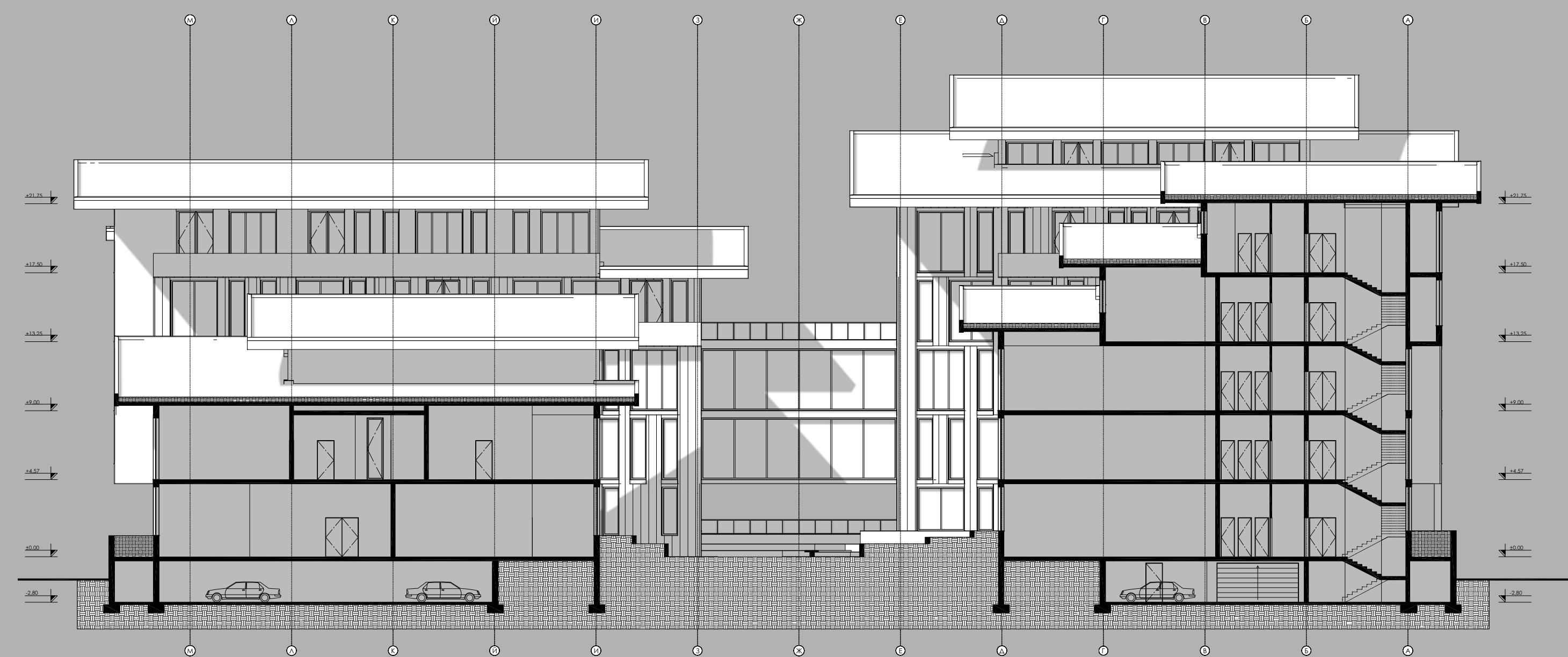
РАЗРЕЗ-S2 М 1:250
