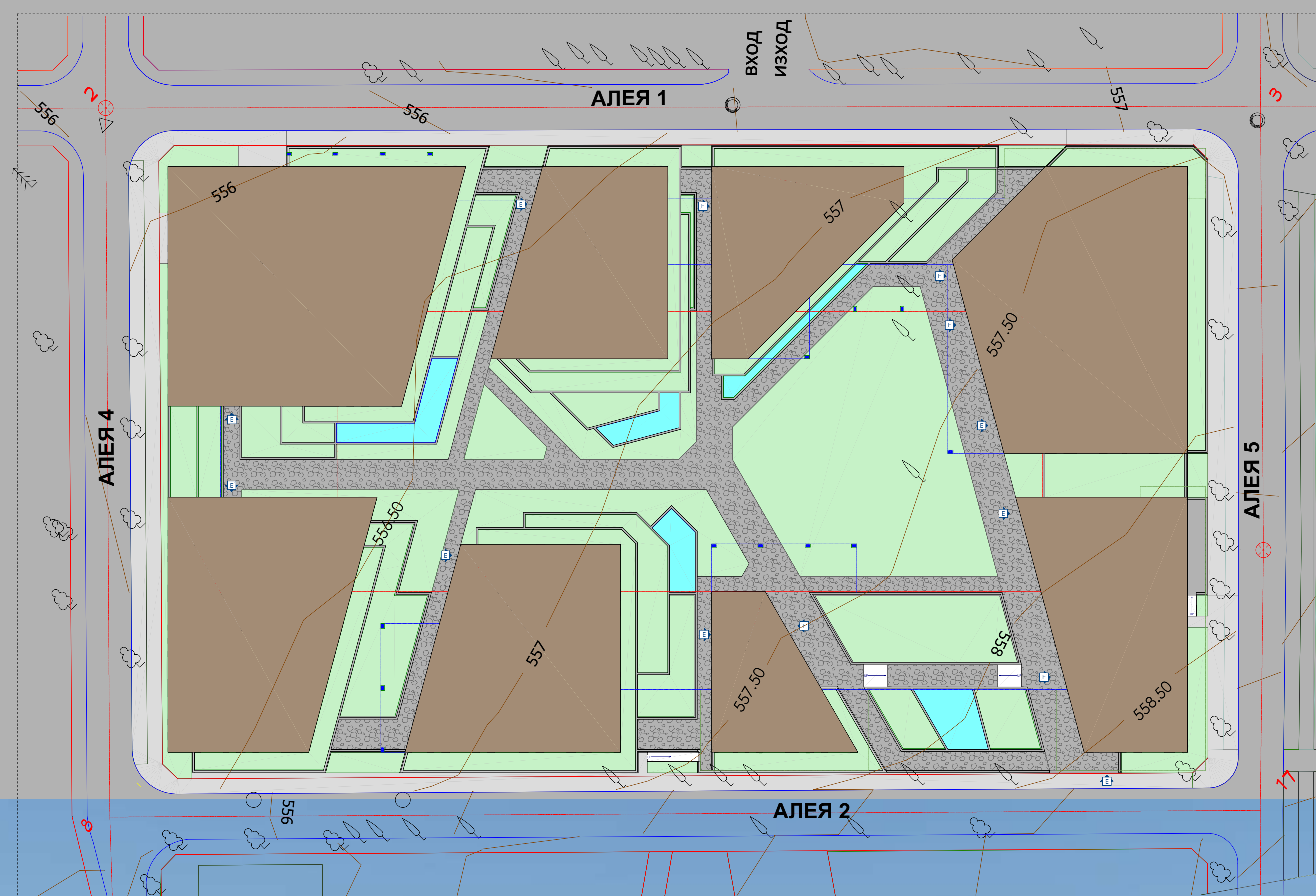
СИТУАЦИЯ М1:500
