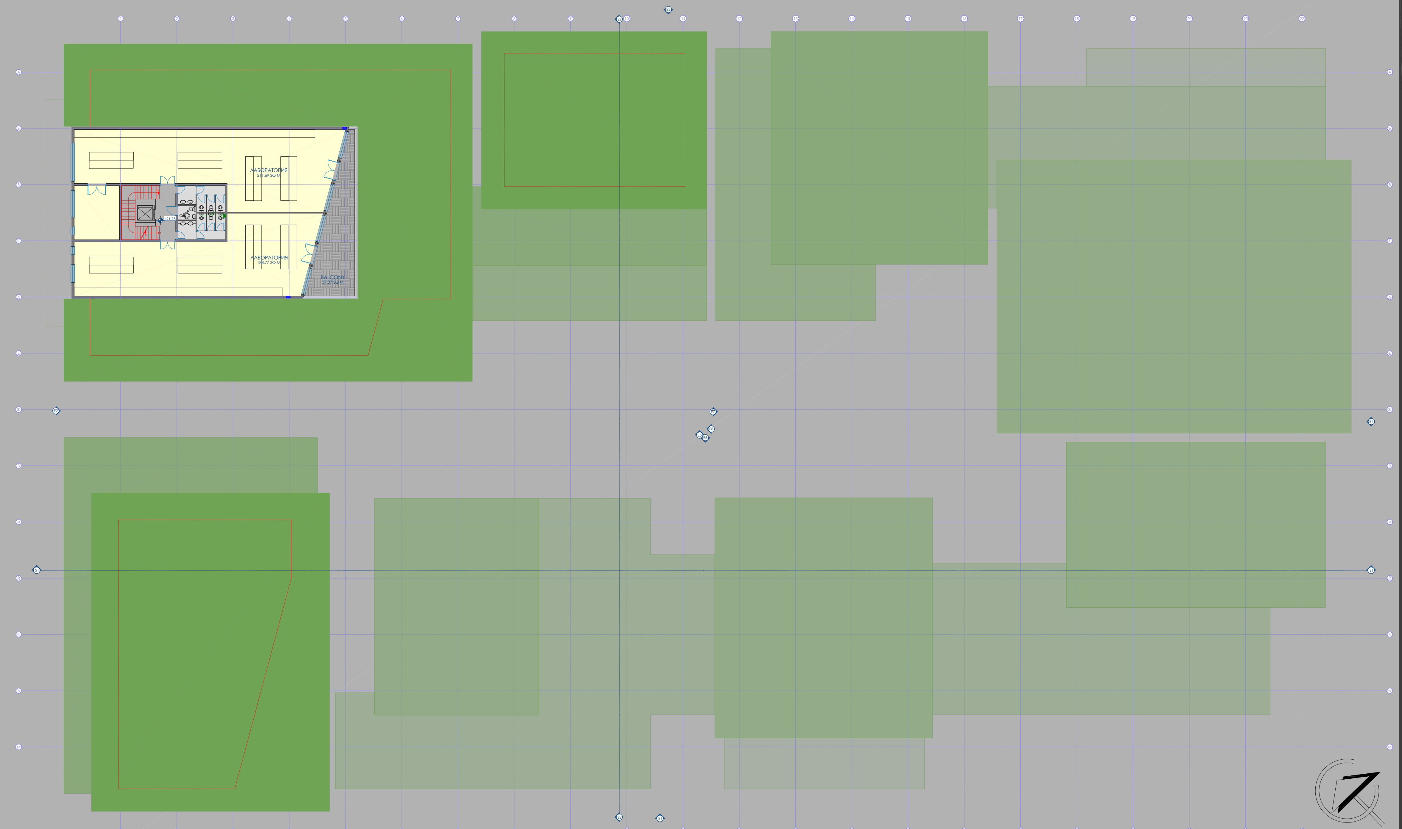
РАЗПРЕДЕЛЕНИЕ НА КОТА+21,75 М 1:250
