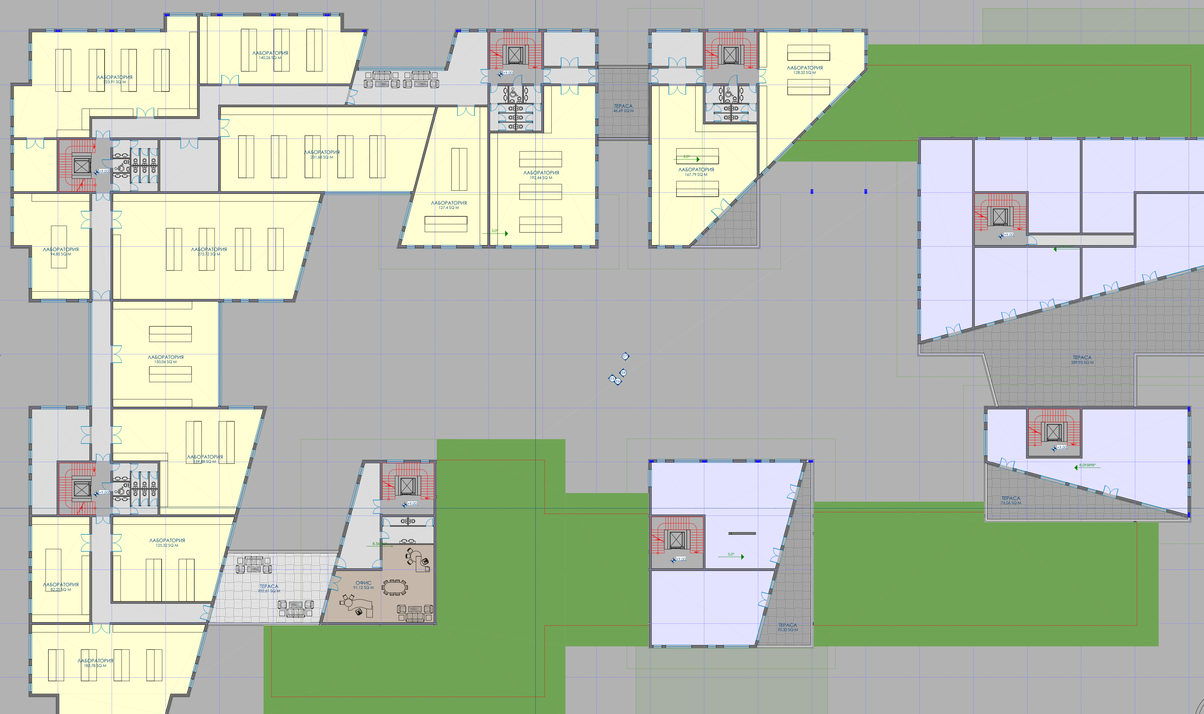
РАЗПРЕДЕЛЕНИЕ НА КОТА+9,00 М 1:250
