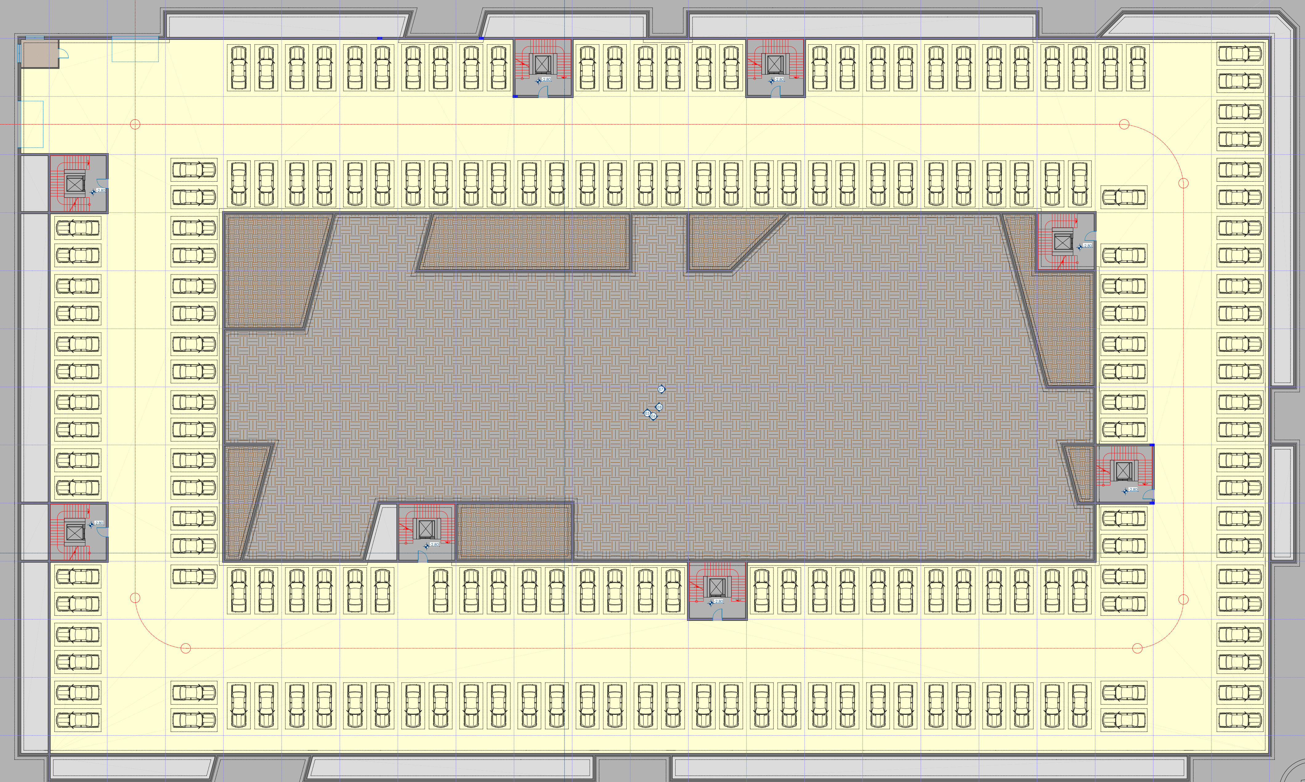
РАЗПРЕДЕЛЕНИЕ НА КОТА-2,80 М 1:250
