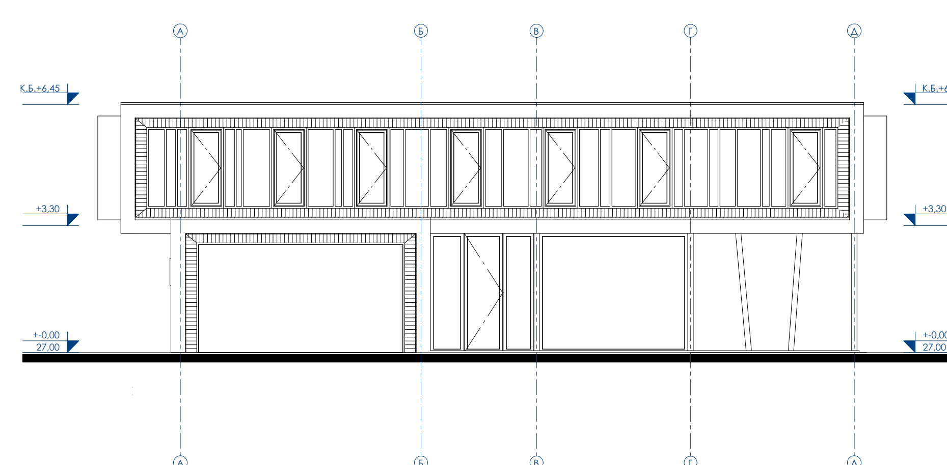
ФАСАДА ЗАПАД М 1:100
