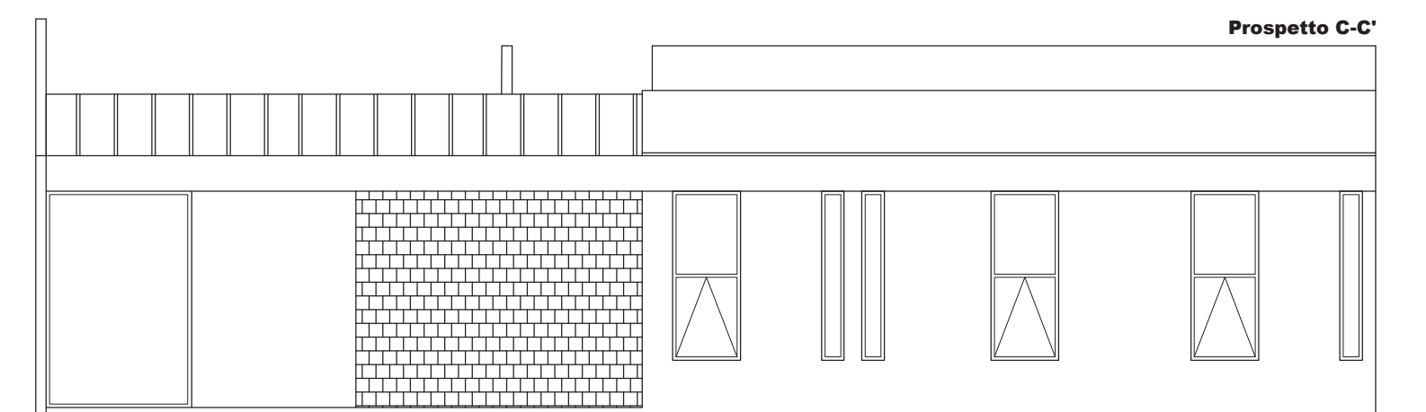
Prospetto C-C'
