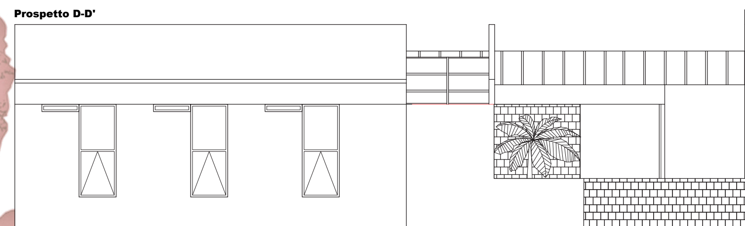
Prospetto D-D'
