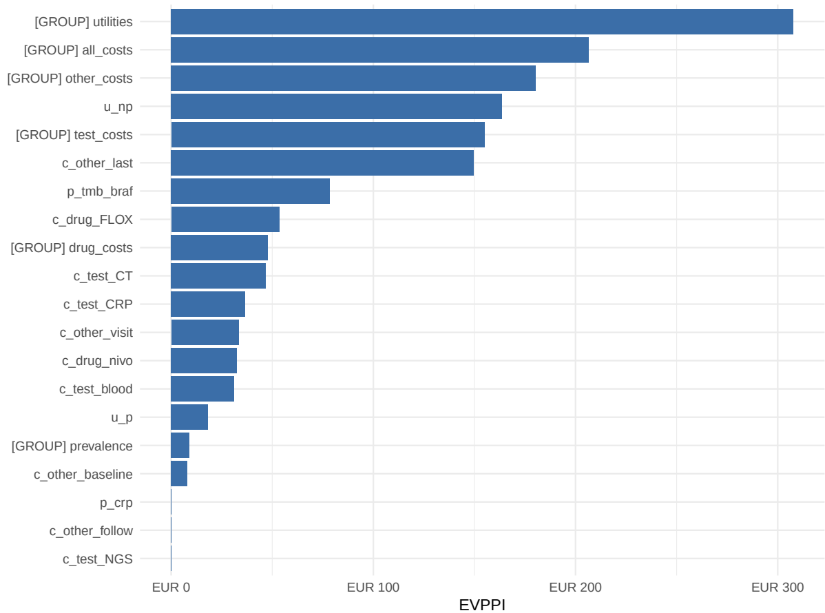
Figure 1: EVPPI by parameter or parameter group
