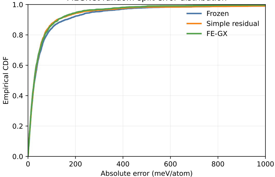
MEGNet random-split error distribution
