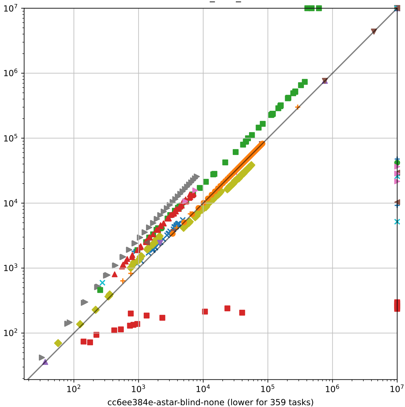
translator_task_size
