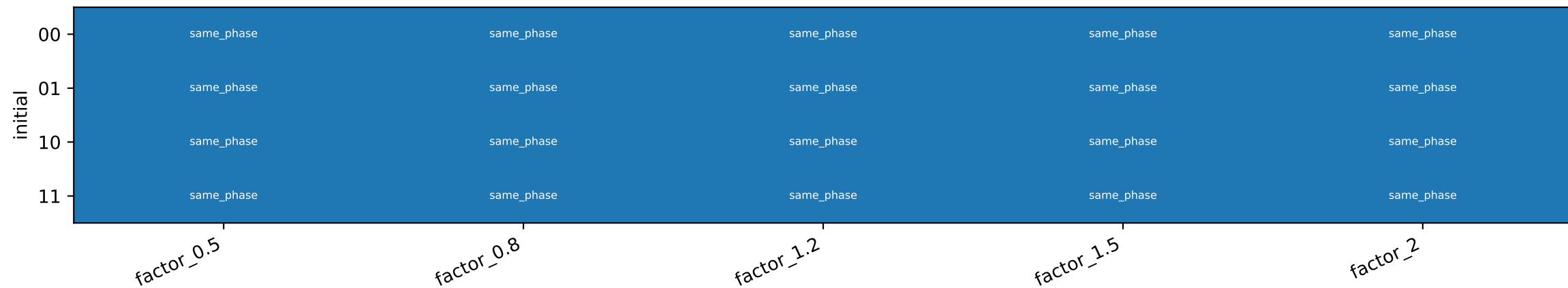
RDF1
