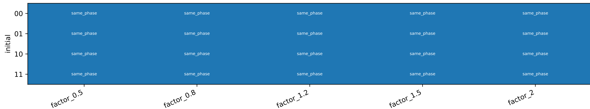
RDF1
