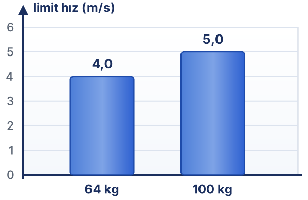
Ş.6 · aynı kubbeyle yapılan iki atlayışın limit hızları
