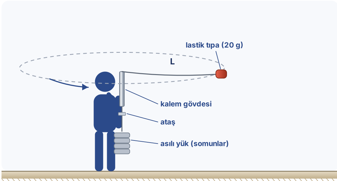
Ş.F1 · düzenek · L, kalem gövdesinin üst ucundan tıpayı kadar olan ip boyudur; ataş, L'nin değişmediğini gösterir
