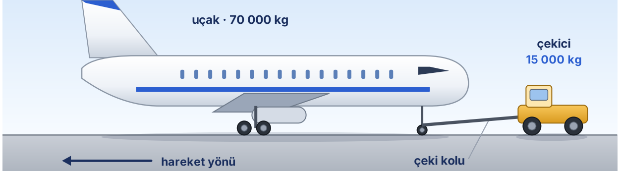
Ş.8 · uçağı çeki koluyla geri iten çekici · ölçekli değildir
