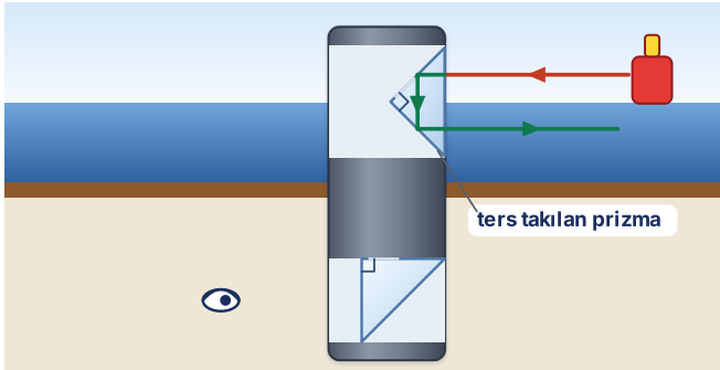
Ş.6 · üst prizması yanlış takılmış periskop
