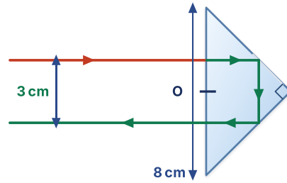
Ş.7 · hipotenüse dik giren ışın · O hipotenüsün orta noktası
