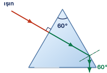
Ş.9 · eşkenar prizma · ışın sol yüze dik giriyor
