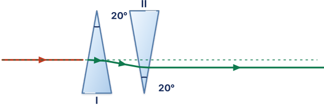
Ş.13 · iki ince prizma · II, I'in ters çevrilmiş hâlidir
