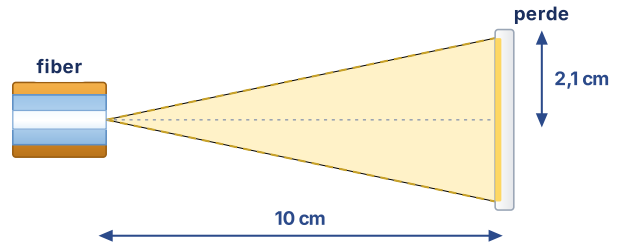
Ş.3 · lifin ucundan çıkan ışığın perdede oluşturduğu daire (yandan görünüş)
