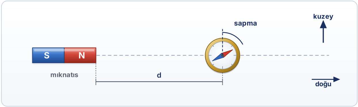
§.8 · üstten görünüş · pusula çubuğun ekseninin uzantısındadır · şekil d = 20 cm durumunu gösterir
