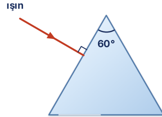
Ş.9 · eşkenar prizma · ışın sol yüze dik giriyor
