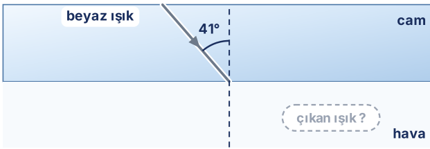
Ş.8 · camın içinden yüzeye gelen beyaz ışık
