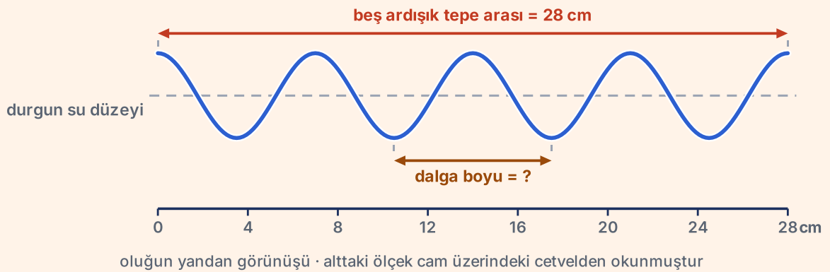
Ş.1 · oluğun yandan görünüşü · durgun su düzeyi kesikli çizgiyle gösterilmiştir
