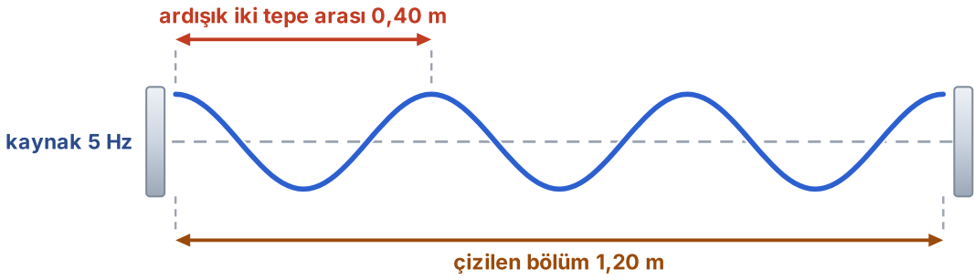
çözgü telinin anlık görüntüsü · telin yalnız üç dalga boyluk bölümü çizilmiştir
