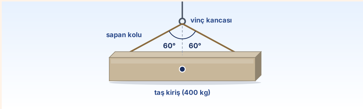
sapanla asılı taş kiriş
