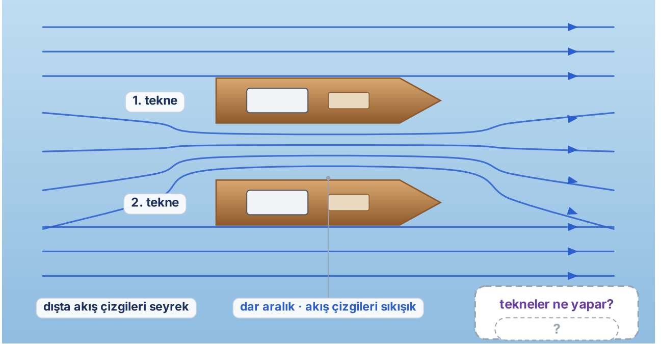
üstten görünüş · iki tekne aynı yöne, birbirine yakın seyreliyor · itilme yönü çizilmemiştir
