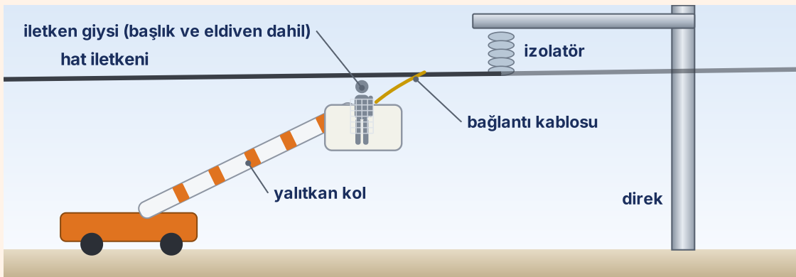
yalıtkan kollu sepetteki çalışan ve hat iletkeni · ölçekli değildir
