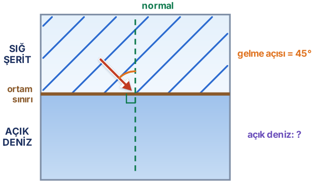
Üstten görünüm · dalga kıyıdan açığa yöneliyor
