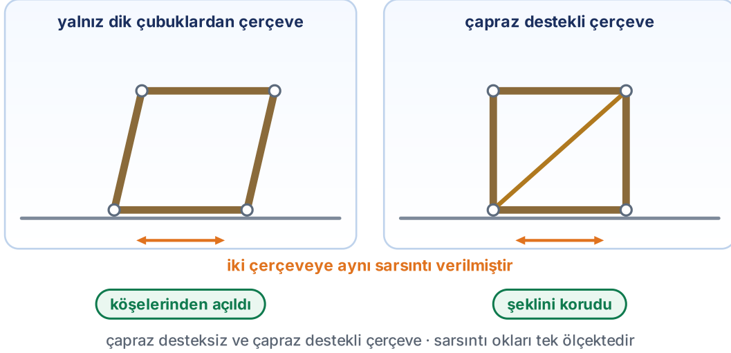
Ş.4 · çapraz desteksiz ve çapraz destekli çerçeve · sarsıntı okları tek ölçektir
