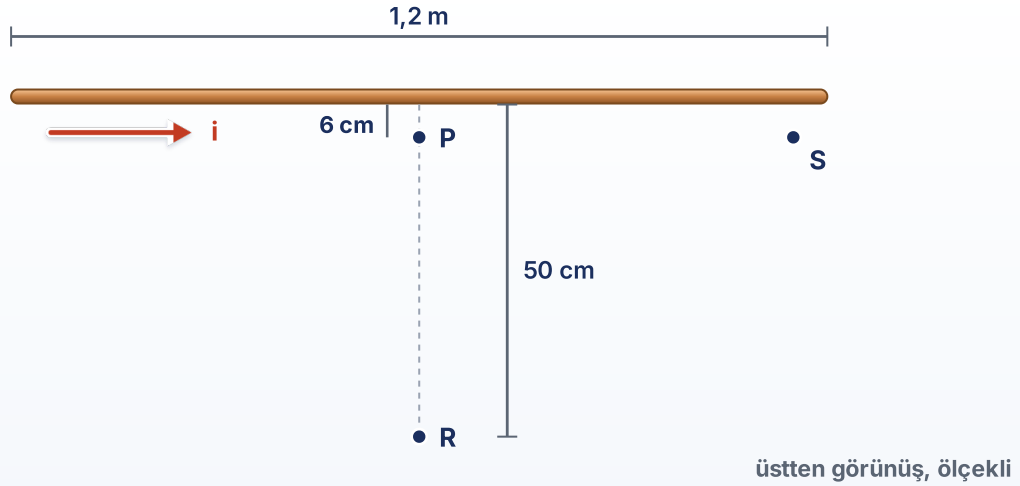
Ş.6 · laboratuvardaki çubuk ve üç ölçüm noktası · P ile S çubuğa 6 cm, R 50 cm uzaktadır · S çubuğun ucundan 5 cm içeridedir
